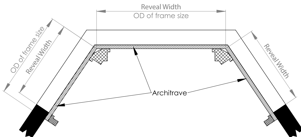
L-FRAME FACE FIT
