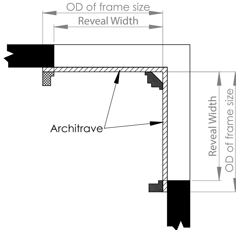
L-FRAME CORNER POST FACE FIT
